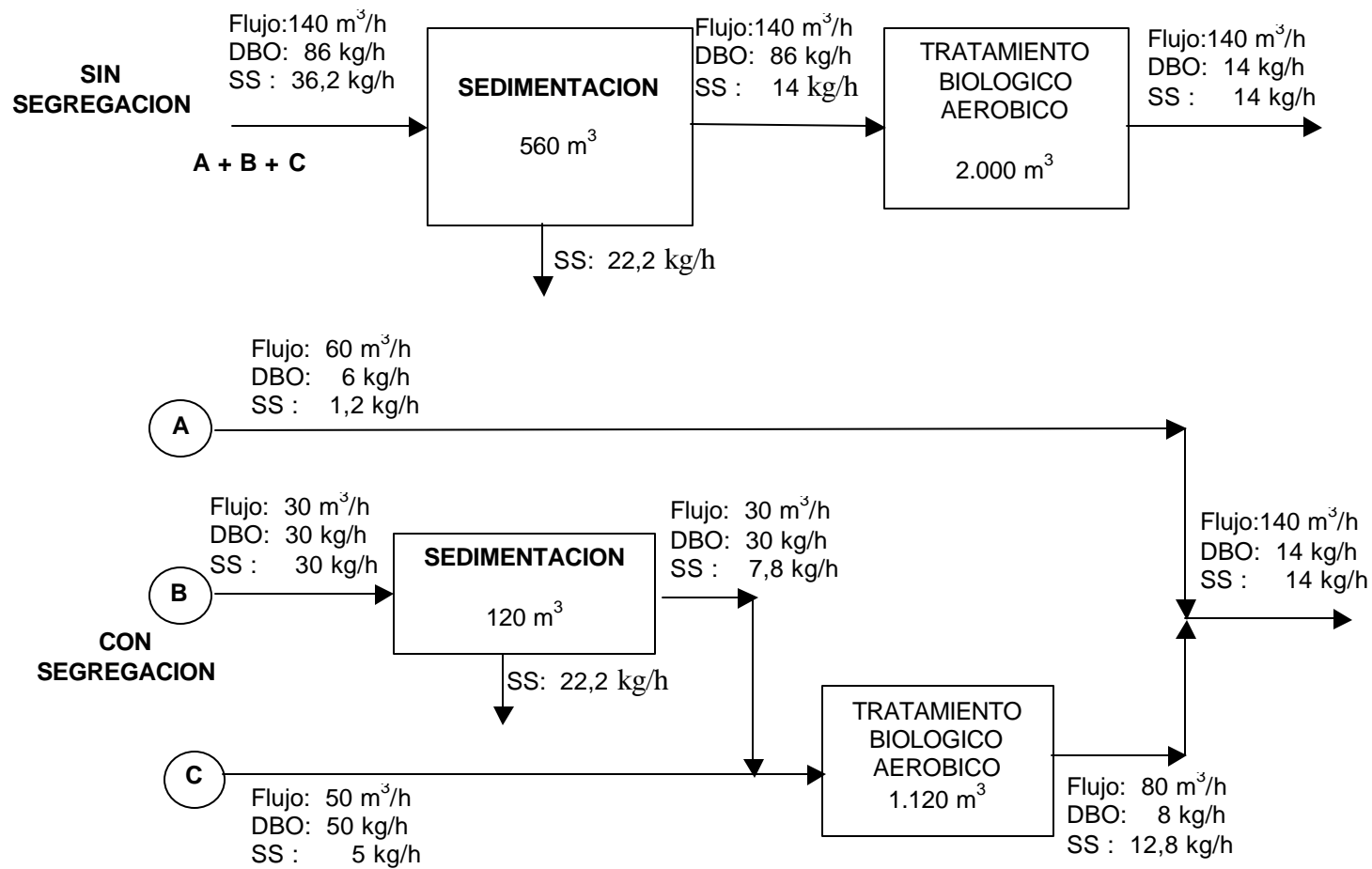
FIGURA 6.6: TRATAMIENTO DIFERENCIADO DE EFLUENTES SEGREGADOS
