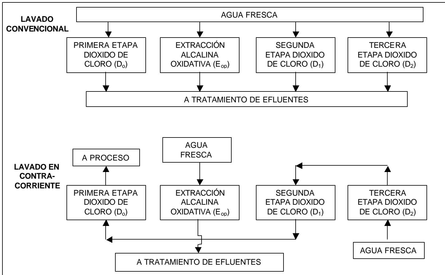
FIGURA 7: SISTEMA DE LAVADO DE PULPA CELULOSICA EN SECUENCIA DE BLANQUEO ECF
