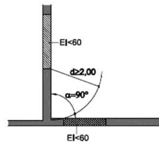
Figura 1.4. Fachadas a 90°
